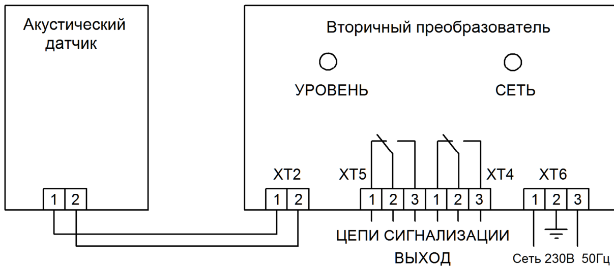
Рисунок В.1 – Схема электрическая подключения регулятора УЗР-1 (не взрывозащищенное исполнение)
