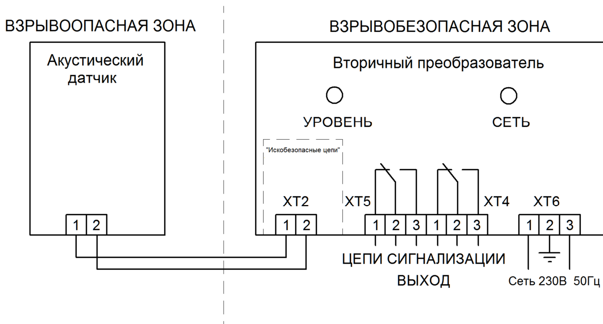
Рисунок В.2 – Схема электрическая подключения регулятора УЗР-1И (взрывозащищенное исполнение)
